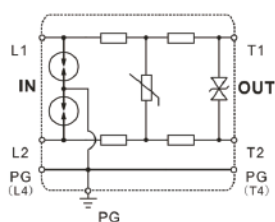
For 1-pair data line DM-...-M2N5
